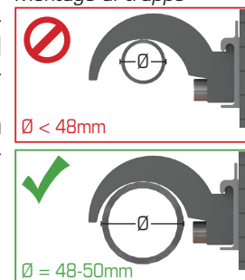
Montage af trappe
